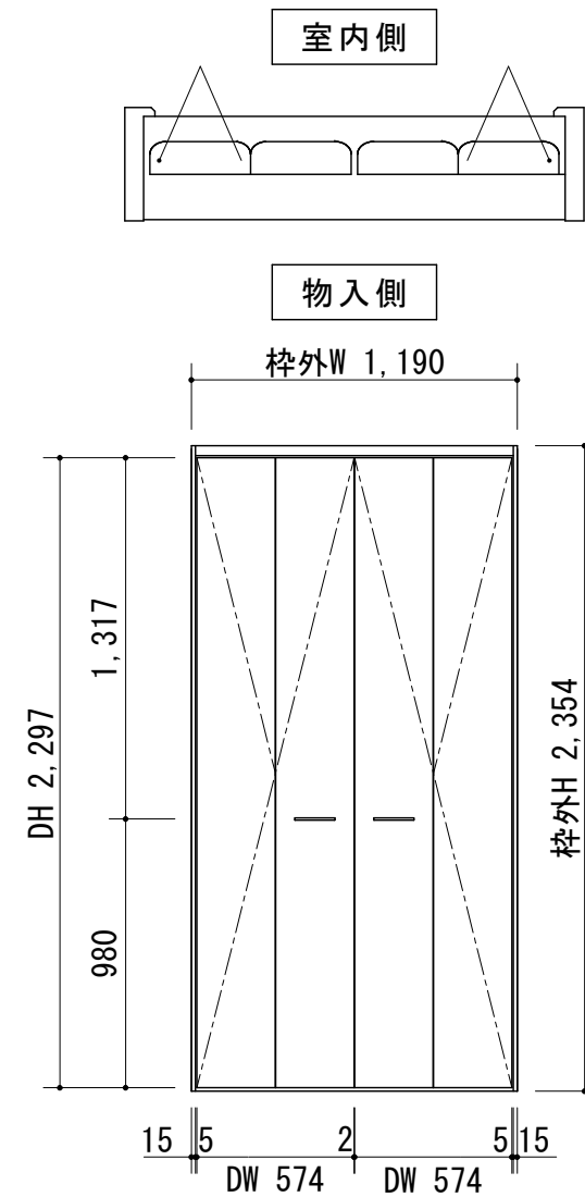
正面図
